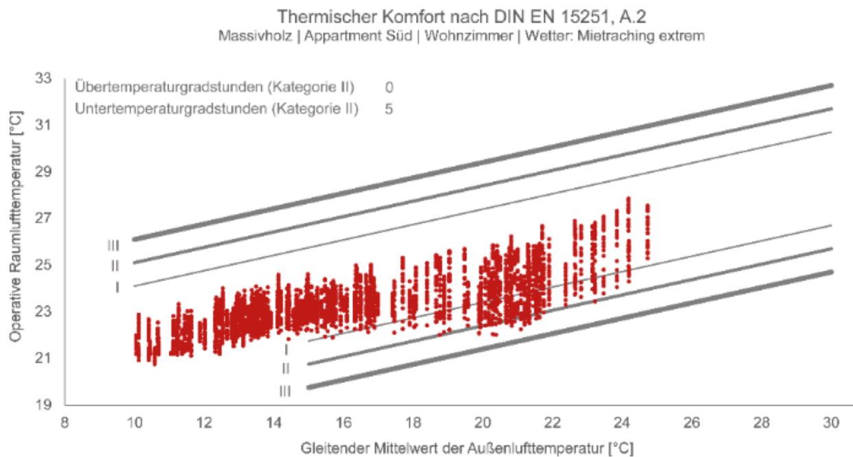
Abbildung 65c: Einfach Bauen 2, DIN EN 15251, Anhang A.2, Thermischer Komfort, Gebäude Holz massiv, Apartment Süd, Wohnzimmer
