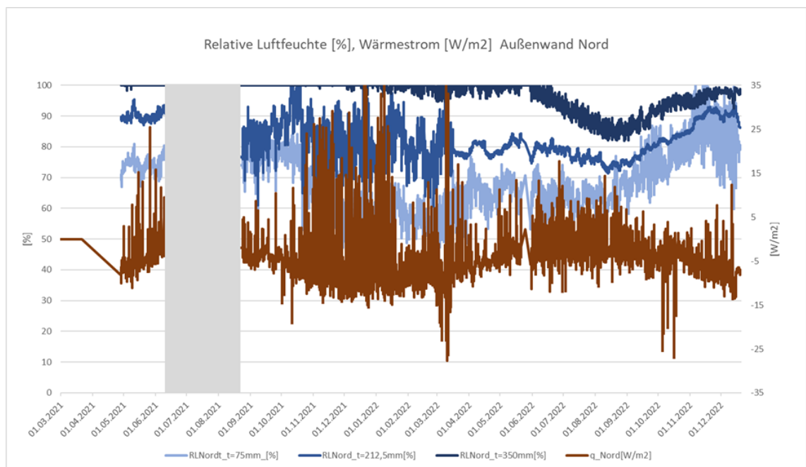
Abbildung 38: relative Luftfeuchte (blau) und Wärmestrom (rot) Nordwand Mauerwerksgebäude, Zsafia Varga
