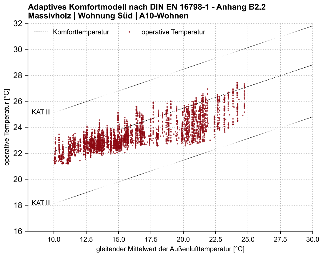
Abbildung 65f: Einfach Bauen 3, DIN EN 16798, Anhang B.2.2, Thermischer Komfort, Gebäude Mauerwerk, Apartment Süd, Wohnzimmer
