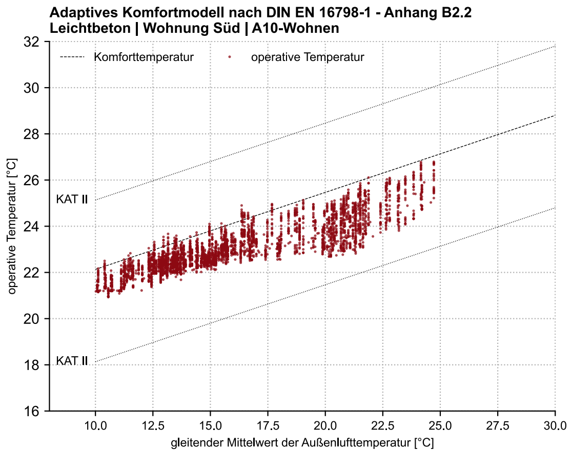
Abbildung 65b: Einfach Bauen 3, DIN EN 16798, Anhang B.2.2, Thermischer Komfort, Gebäude Leichtbeton, Apartment Süd, Wohnzimmer
