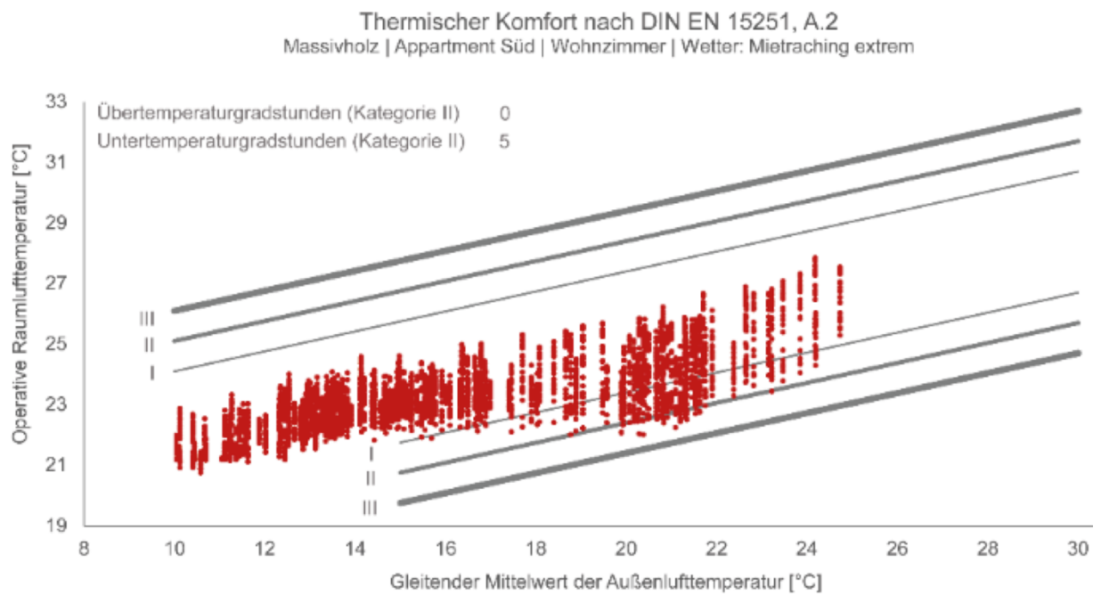
Abbildung 65e: Einfach Bauen 2, DIN EN 15251, Anhang A.2, Thermischer Komfort, Gebäude Mauerwerk, Apartment Süd, Wohnzimmer
