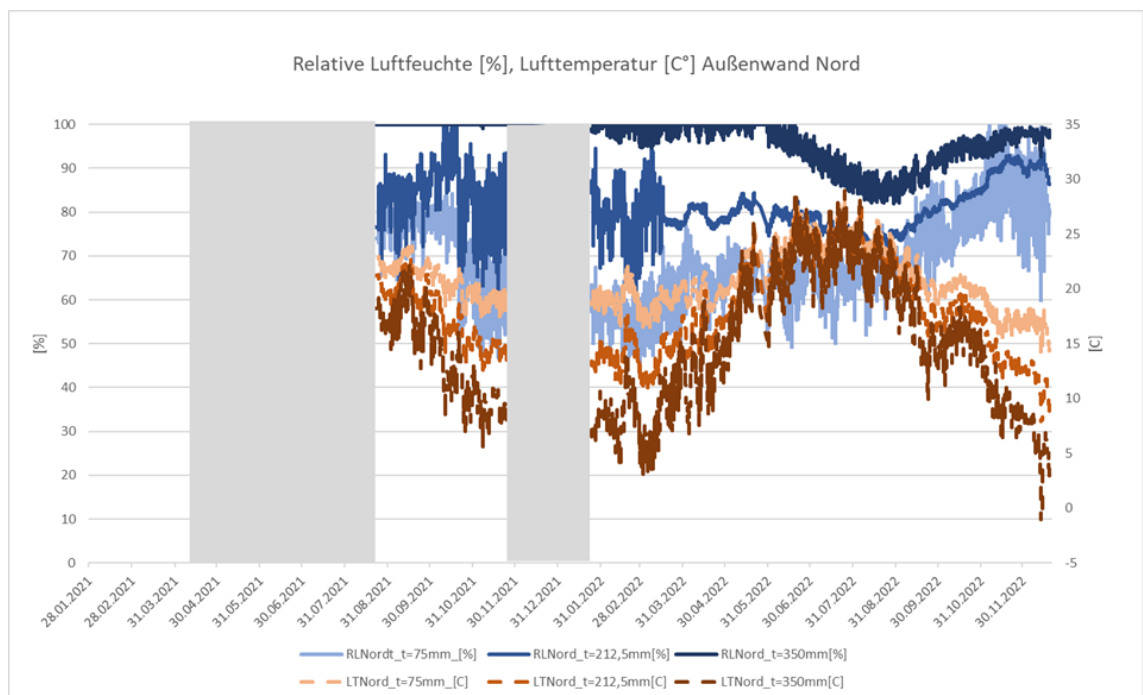
Abbildung 34: relative Luftfeuchte (blau) und Lufttemperatur (rot) Nordwand Mauerwerksgebäude, Zsafia Varga
