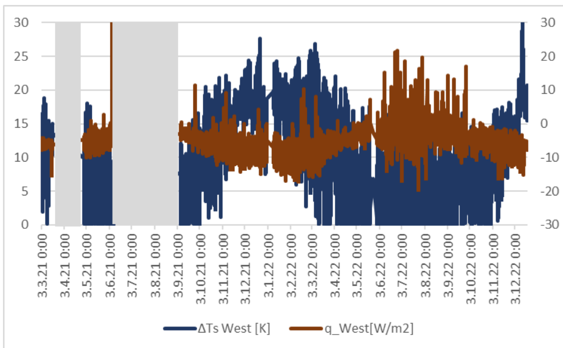
Abbildung 21: Temperaturunterschied Oberfläche Ts und Wärmestrom q Westwand, Mauerwerksgebäude, Zsafia Varga
