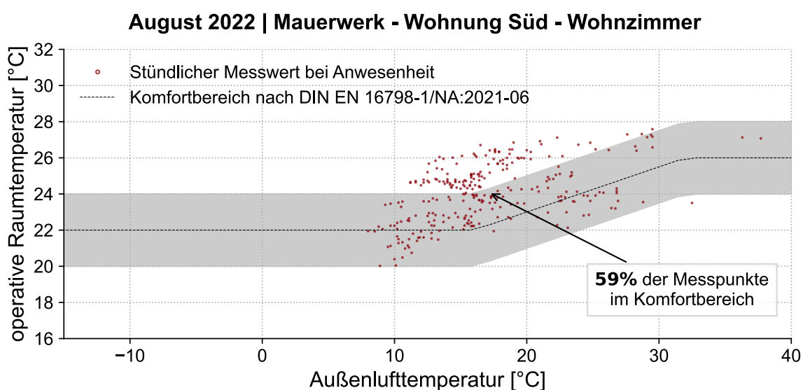
Abbildung 83: Thermischer Komfort (operative Temperatur), August 2022, Mauerwerk Süd, Wohnzimmer
