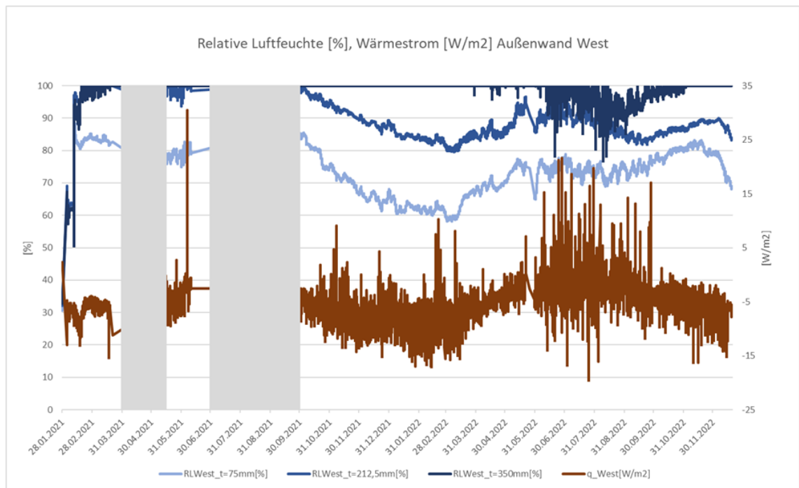
Abbildung 37: relative Luftfeuchte (blau) und Wärmestrom (rot) Westwand Mauerwerksgebäude, Zsafia Varga
