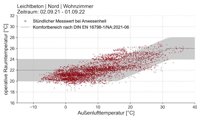
Abbildung 53: Thermischer Komfort – 2. OG | Wohnung Nord | Wohnzimmer
