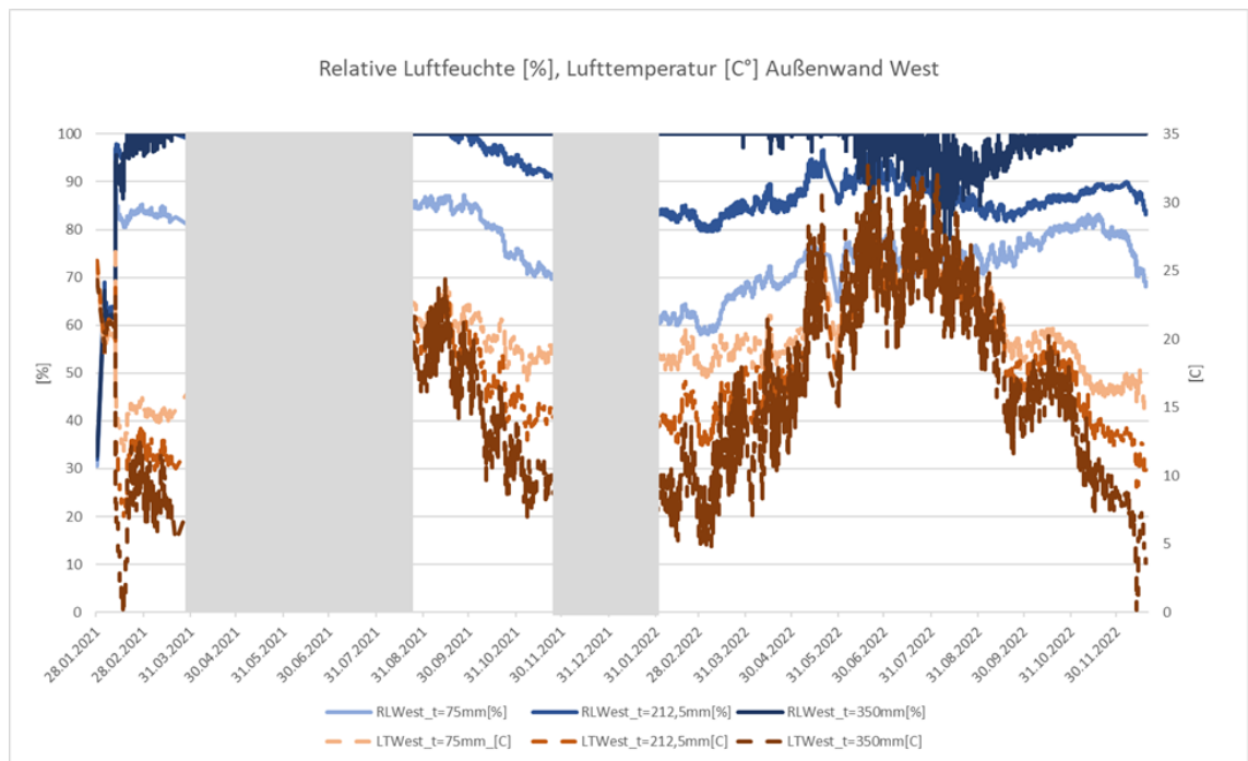
Abbildung 33: relative Luftfeuchte (blau) und Lufttemperatur (rot) Westwand Mauerwerksgebäude, Zsafia Varga
