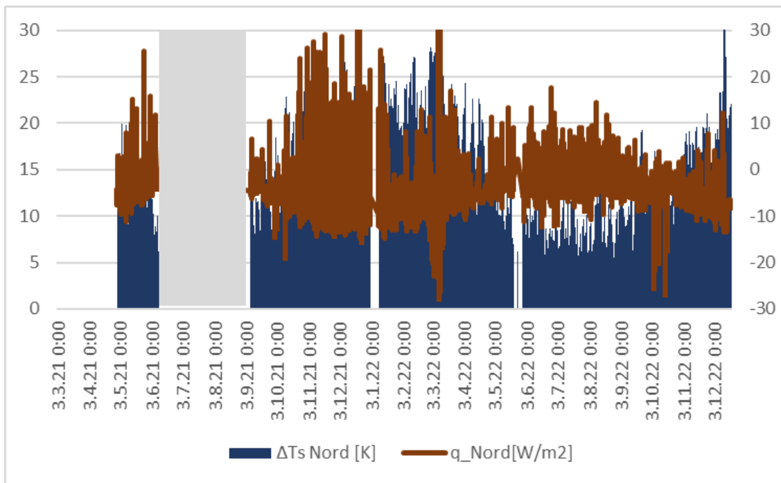
Abbildung 20: Temperaturunterschied Oberfläche Ts und Wärmestrom q Nordwand, Mauerwerksgebäude, Zsafia Varga
