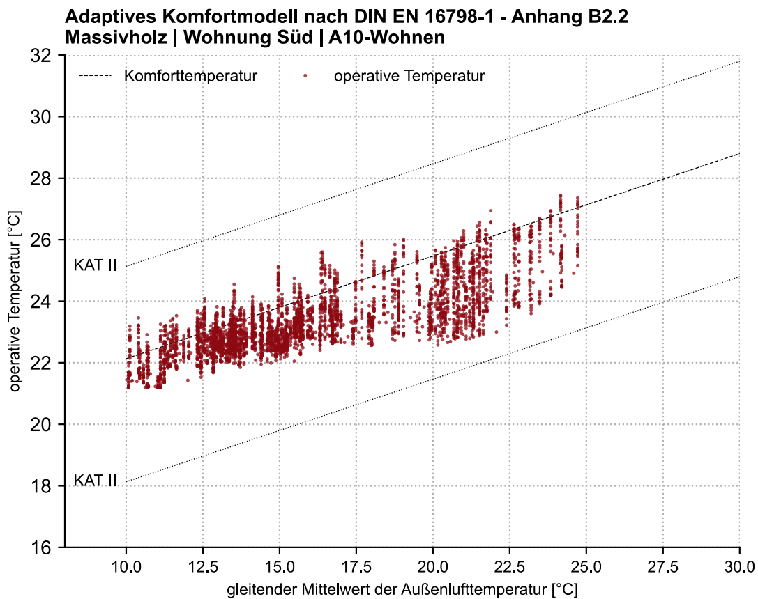
Abbildung 65d: Einfach Bauen 3, DIN EN 16798, Anhang B.2.2, Thermischer Komfort, Gebäude Holz massiv, Apartment Süd, Wohnzimmer
