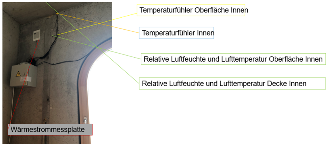
Abbildung 10: Aufbau Messtechnik Westseite Leichtbetongebäude
