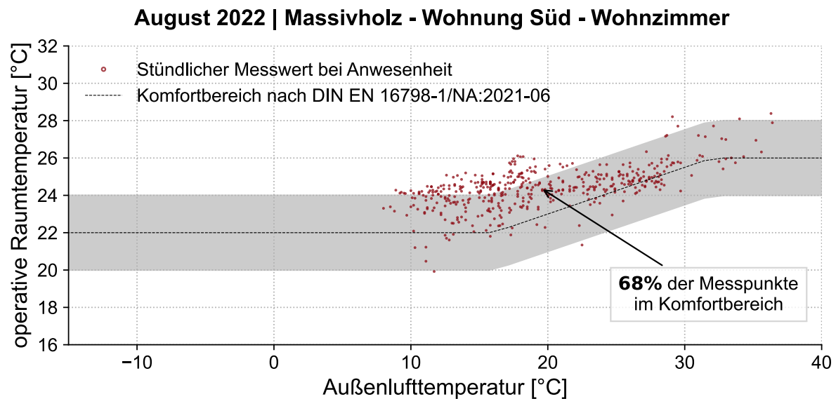
Abbildung 82: Thermischer Komfort (operative Temperatur), August 2022, Massivholz Süd, Wohnzimmer
