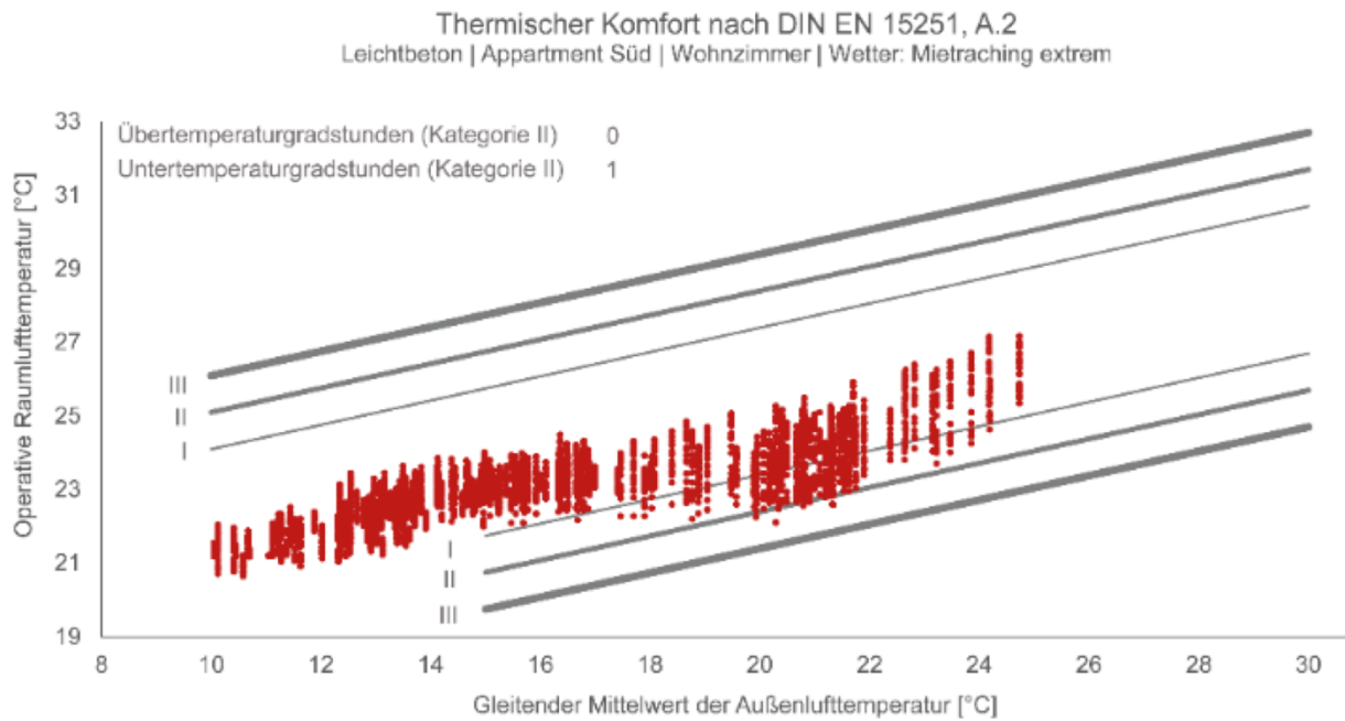
Abbildung 65a: Einfach Bauen 2, DIN EN 15251, Anhang A.2, Thermischer Komfort, Gebäude Leichtbeton, Apartment Süd, Wohnzimmer
